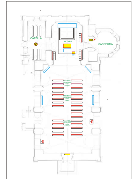
RISCALDAMENTO A RADIATORE CERAMICO TERMO-RAD-HORIZON
